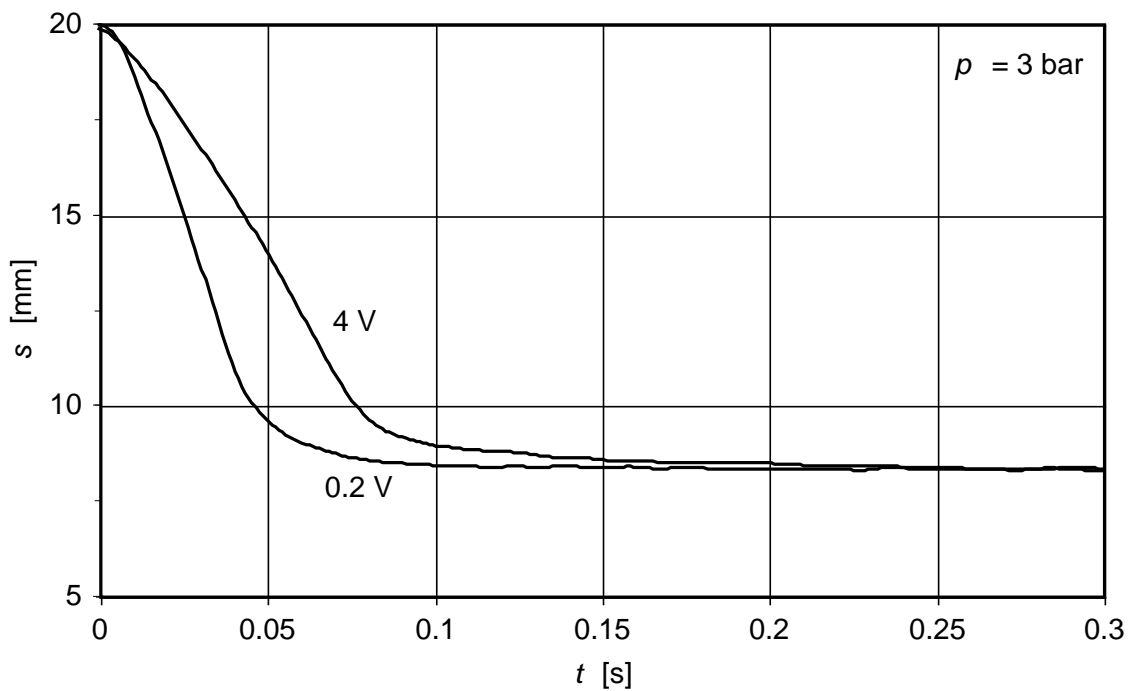
Bild 6: Verlauf des Greifvorganges bei verschiedenen Drosselstellungen ( U_R = 0.2 \text{ V} bzw. U_R = 4 \text{ V} ) für Kabelbaum CF
